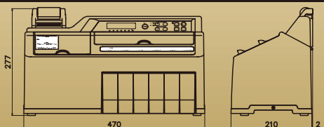
寸 法 図
